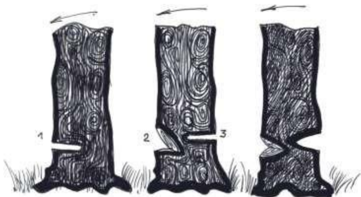
Рис. 9. Черговість запилів (1, 2) та підрубів (3) при рубанні
